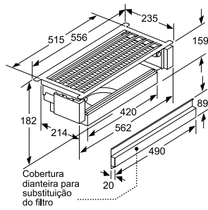
Instalação do exaustor integrável com módulo cleanAir
