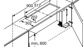
Instalação do exaustor telescópico com módulo cleanAir
