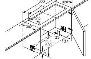
Instalação do exaustor telescópico com módulo cleanAir
