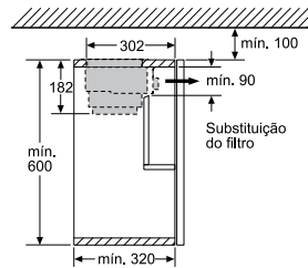
Instalação do exaustor integrável com módulo cleanAir
