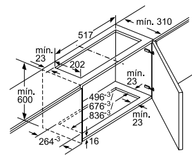
Instalação da caixa do ventilador com módulo cleanAir
